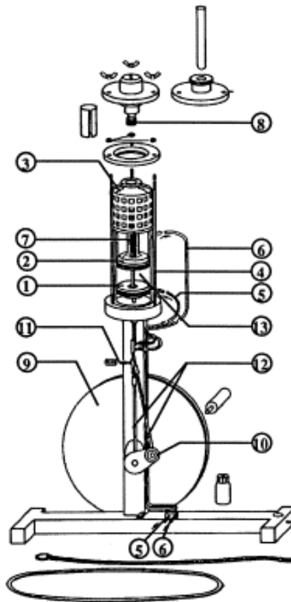
Figur 4. Den Stirlingmotor som du ska använda under laborationen.
