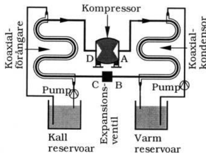
Figur 6. Värmepumpsanläggning med koaxialförångare och koaxialkondensor.
